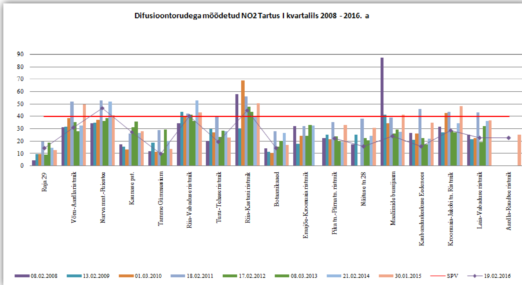
Joonis 4. Difusioonitorudega mõõdetud NO 2 Tartus I kvartalis 2008-2016.a.
