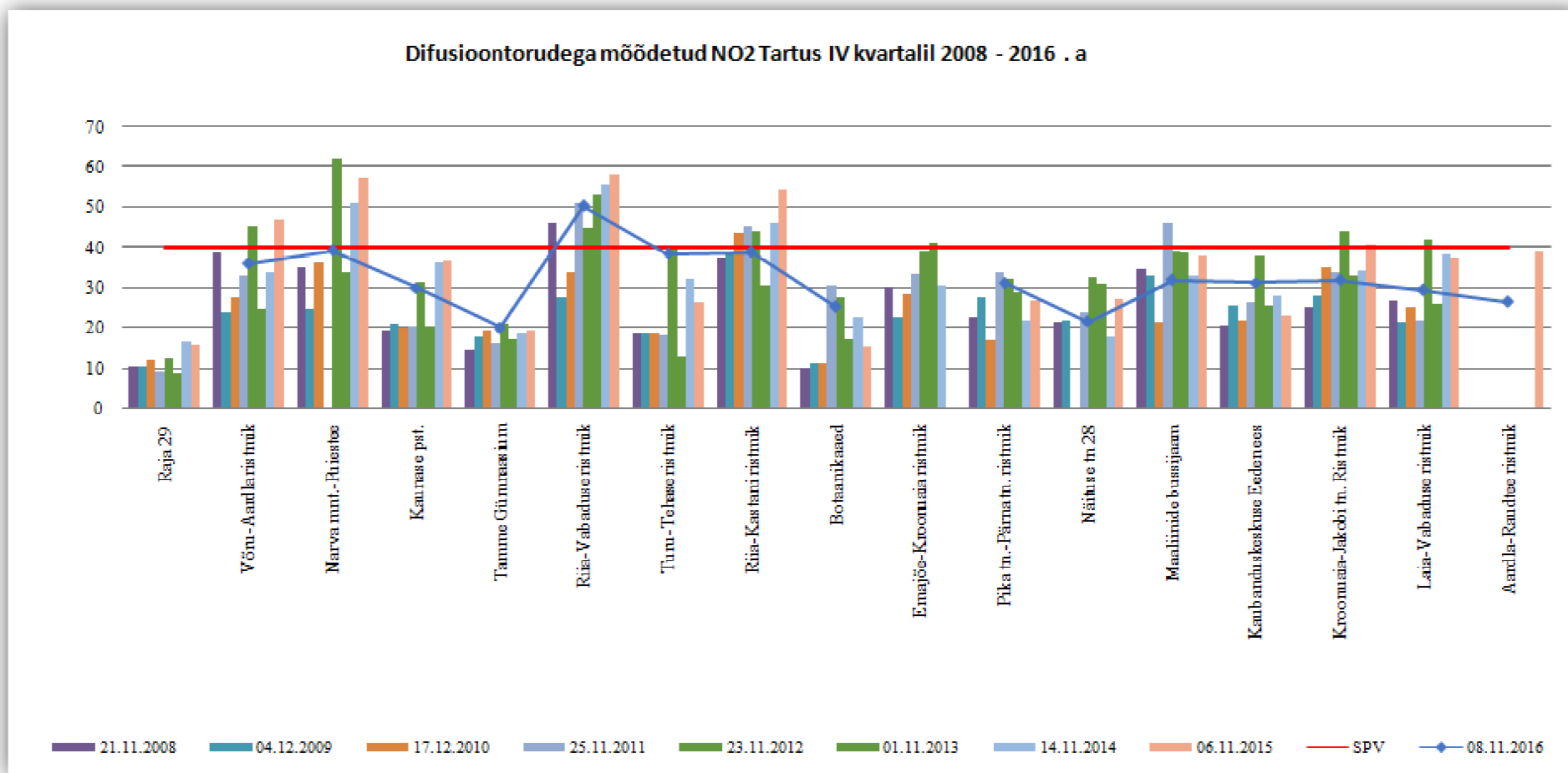
Joonis 7. Difusioontorudega mõõdetud NO 2 Tartus IV kvartalis 2008-2016.a.
