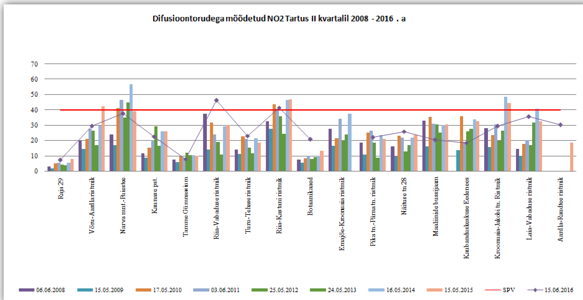
Joonis 5. Difusioonitorudega mõõdetud NO 2 Tartus II kvartalis 2008-2016.a.
