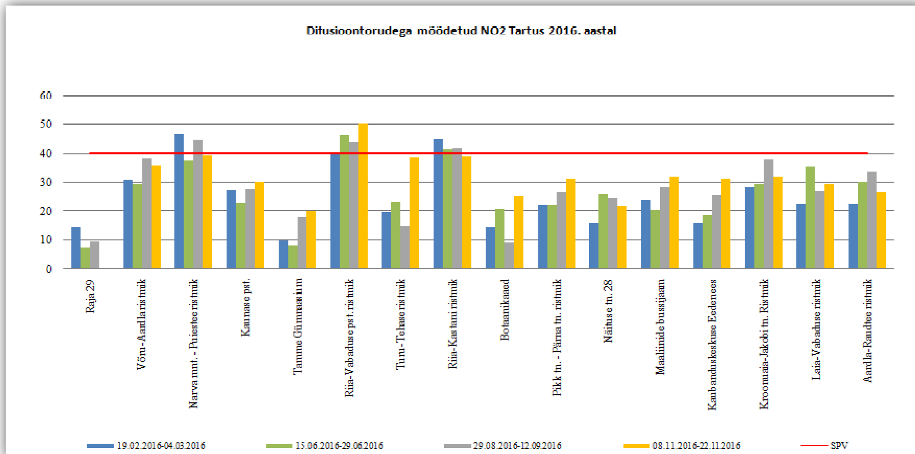
Joonis 3. Difusioontorudega mõõdetud NO 2 Tartus 2016.aastal
