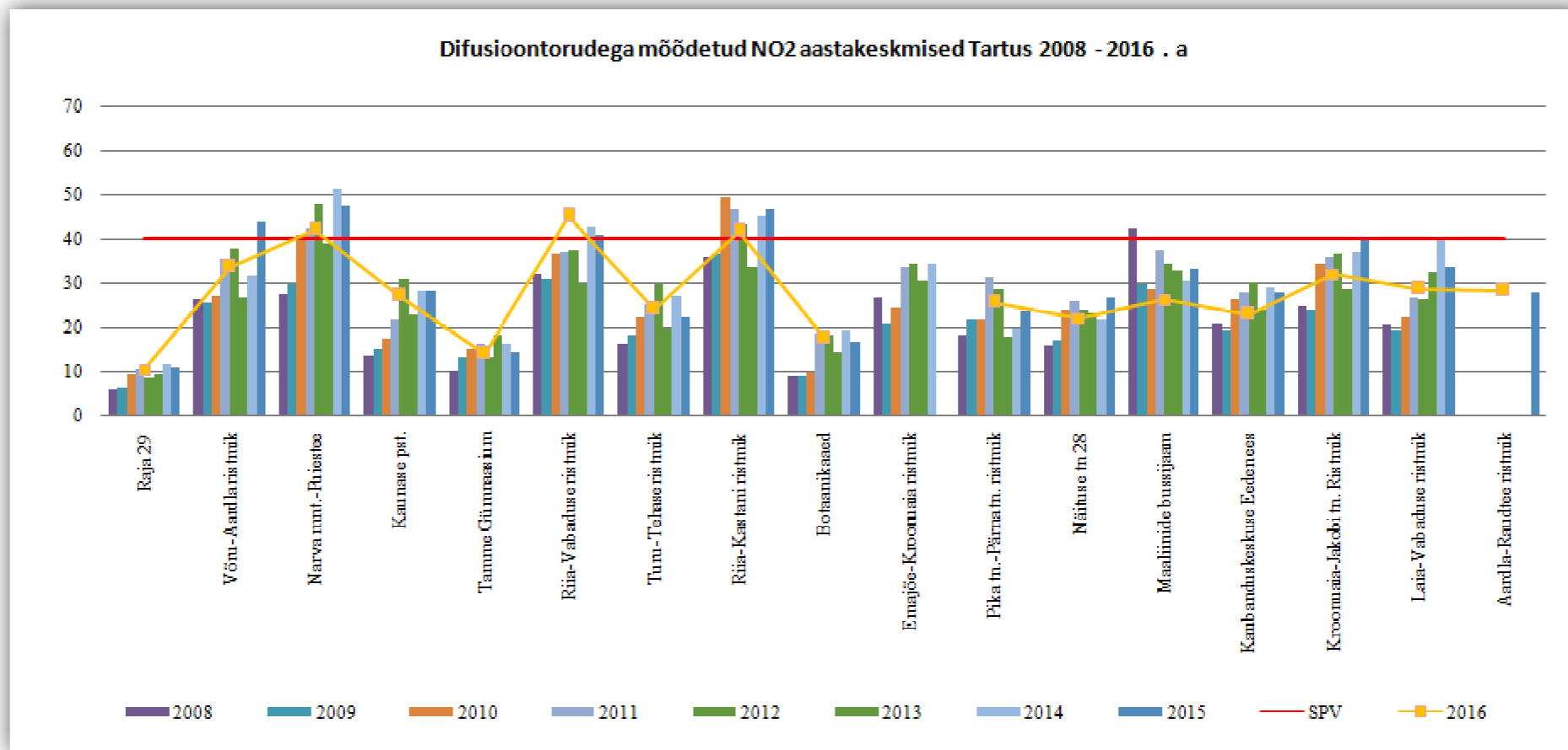
Joonis 8. Difusioonitorudega mõõdetud NO 2 Tartus, aastakeskmised kontsentratsioonid 2008-2016.a.
