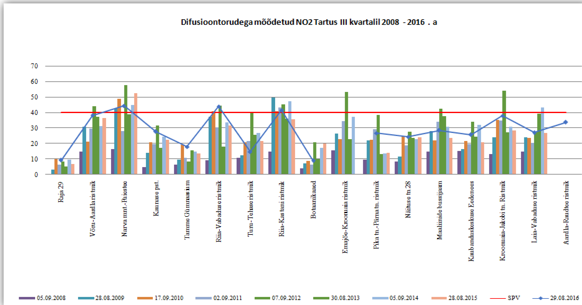
Joonis 6. Difusioontorudega mõõdetud NO 2 Tartus III kvartalis 2008-2016.a.
