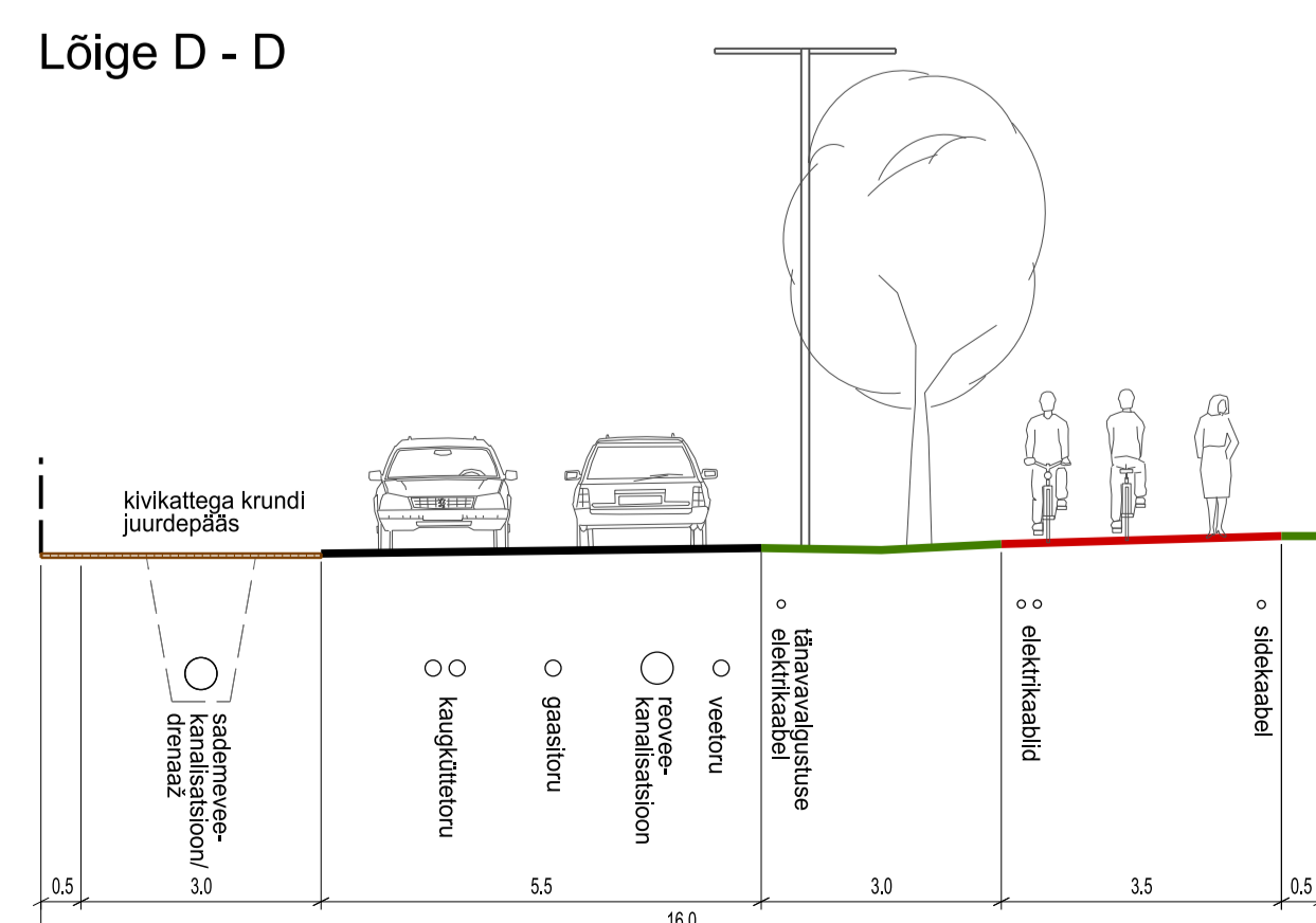
Lõige D - D
