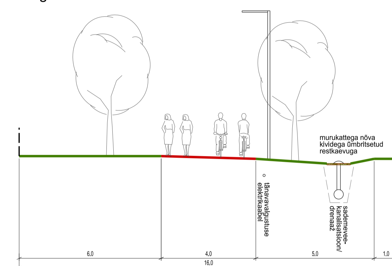
Lõige B - B
