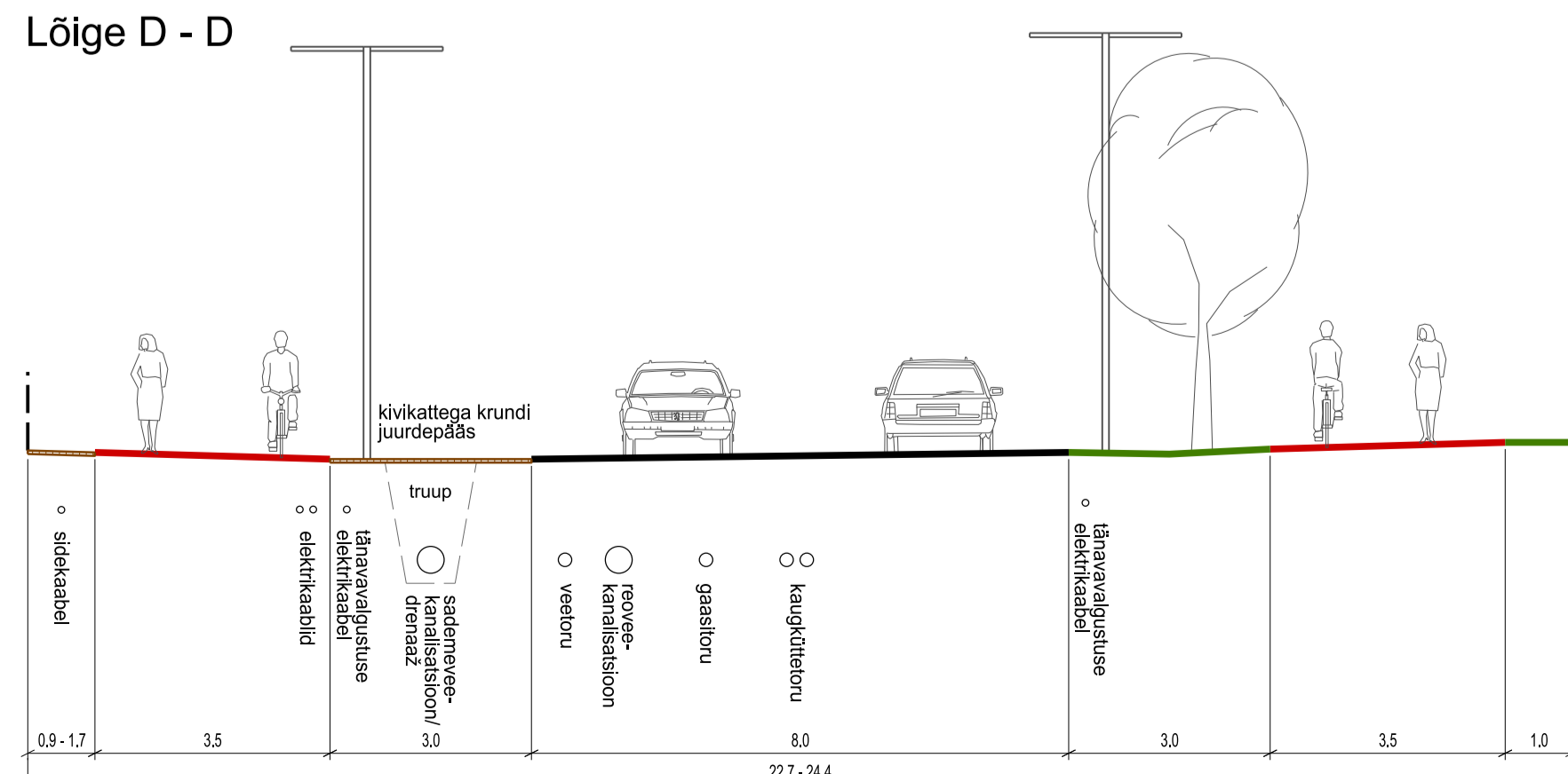
Lõige D - D
