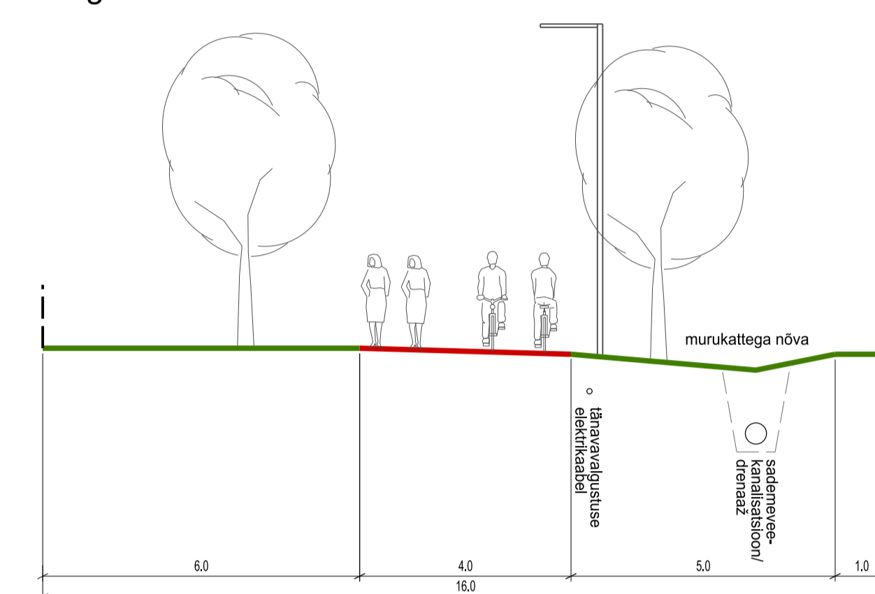
Lõige A - A
