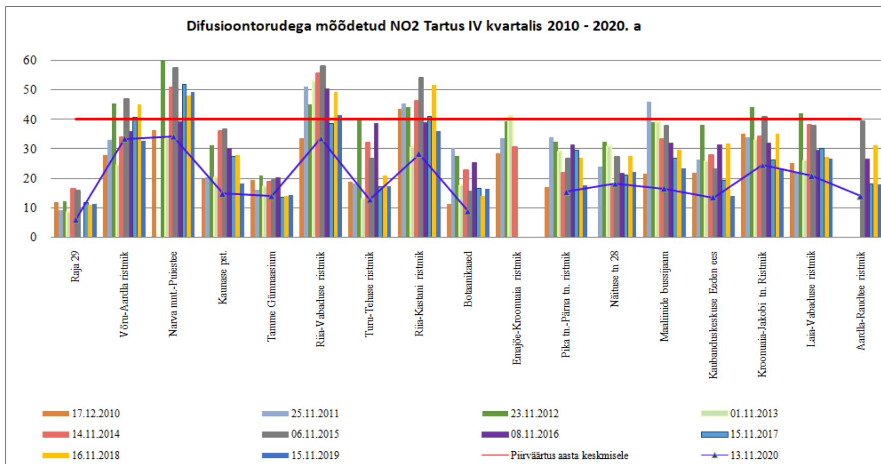
Joonis 7. Difusioontorudega mõõdetud NO 2 Tartus IV kvartalis 2010-2020. a.
