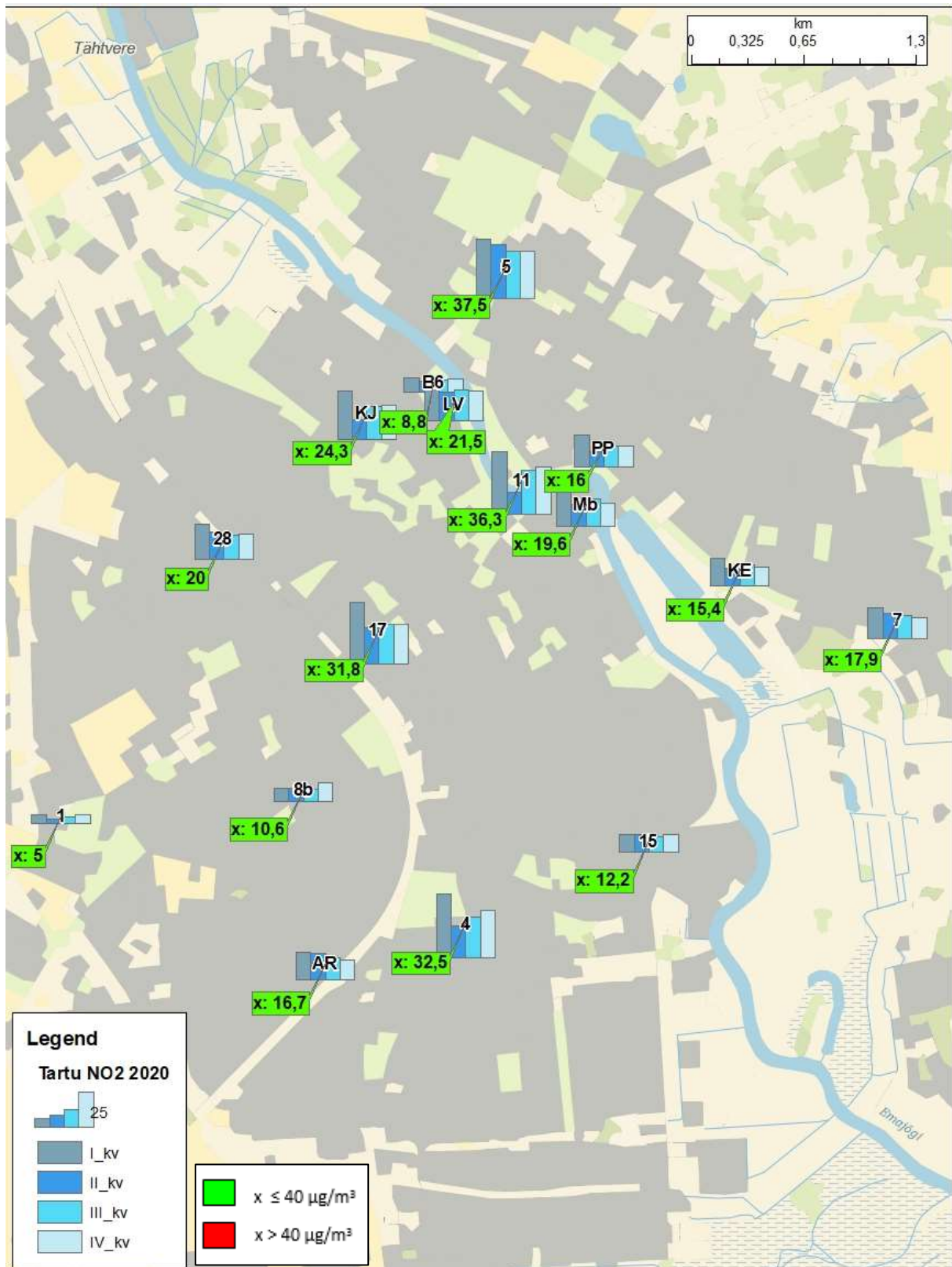
Joonis 2. Tartu linna 2020. aasta välisõhu saasteaine NO 2 kontsentratsioonid I, II, III ja IV kvartalis, 2020. aasta keskmine x (Nr diagrammil on seirejaama tähis)
