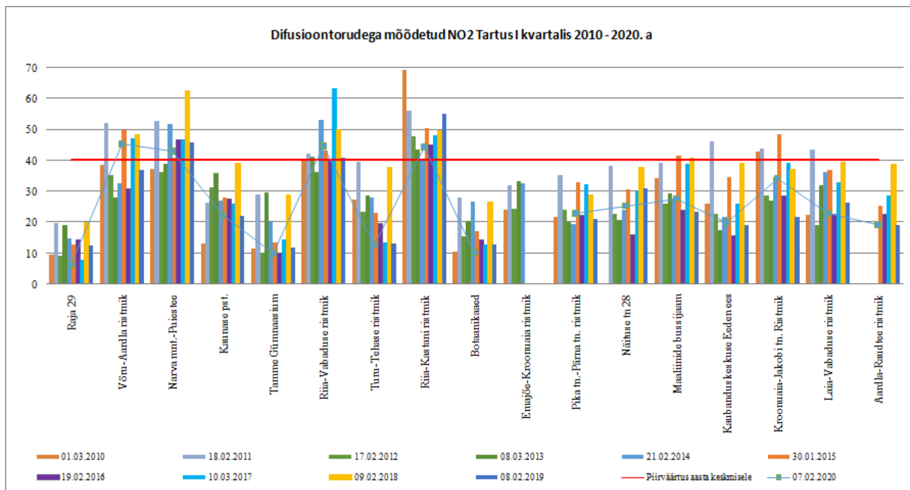
Joonis 4. Difusioontorudega mõõdetud NO 2 Tartus I kvartalis 2010-2020 a.
