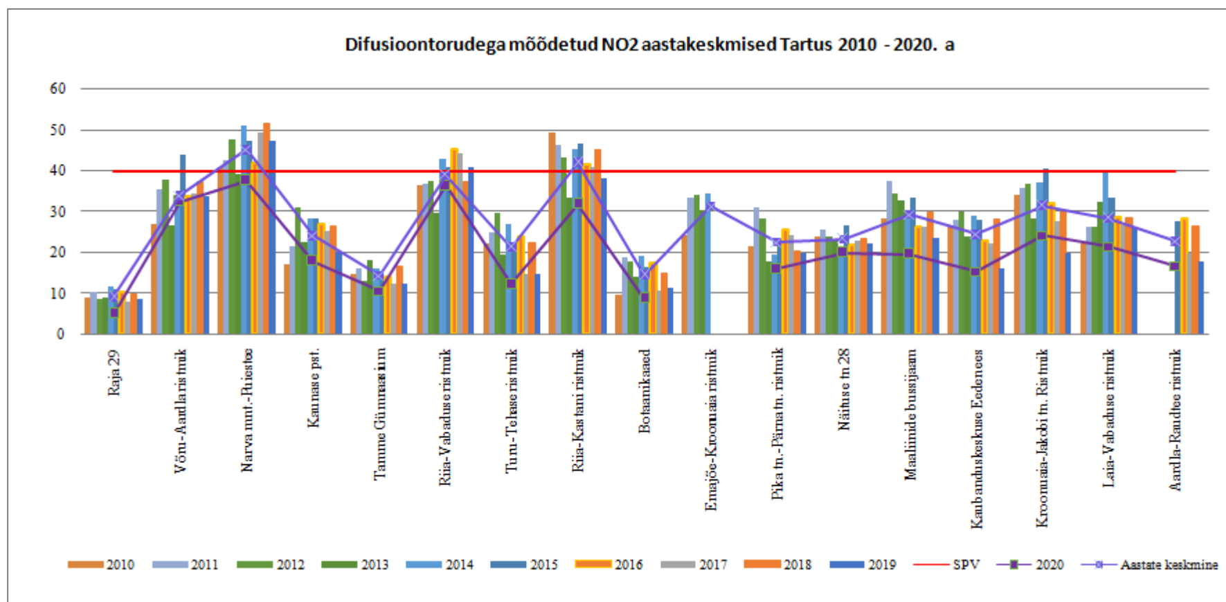
Joonis 8. Difusioonitorudega mõõdetud NO 2 Tartus, aastakeskmised kontsentratsioonid 2010-2020.a.
