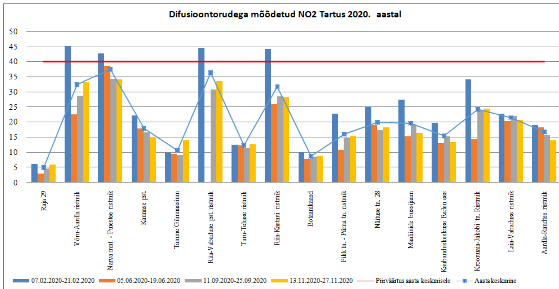
Joonis 3. Difusioonitorudega mõõdetud NO 2 Tartus 2020. aastal
