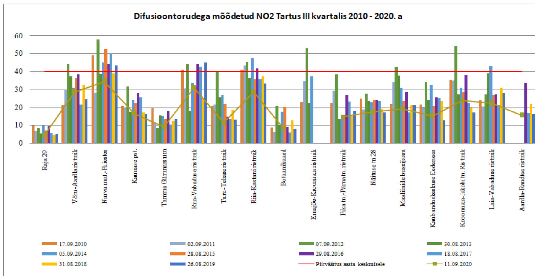
Joonis 6. Difusioonitorudega mõõdetud NO 2 Tartus III kvartalis 2010-2020. a.
