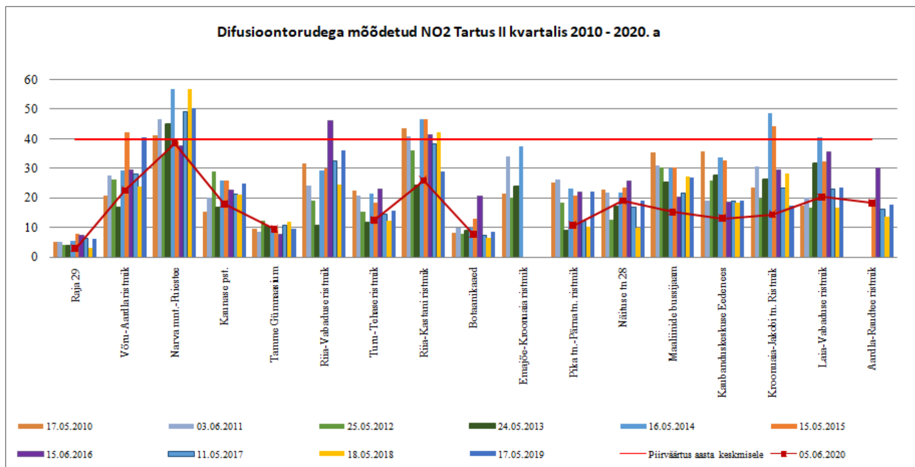
Joonis 5. Difusioontorudega mõõdetud NO 2 Tartus II kvartalis 2010-2020 a.
