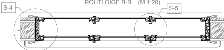
RÕHTLÕIGE B-B (M 1:20)
