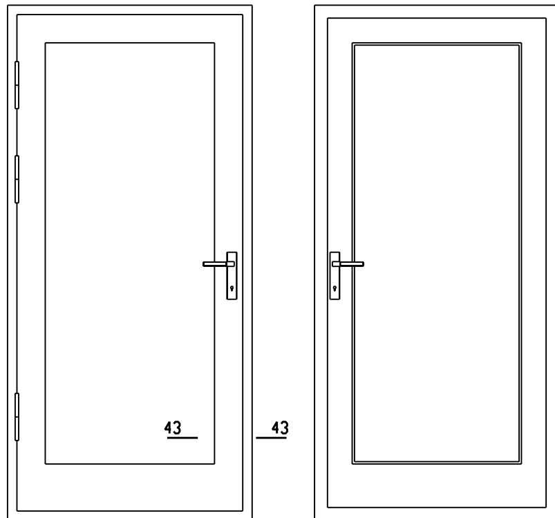
Vaade väljast m1:20
