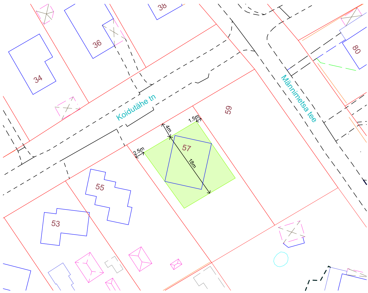
Lisa. Koidutähe tn 57 ehitusala skeem PTH-24-067
