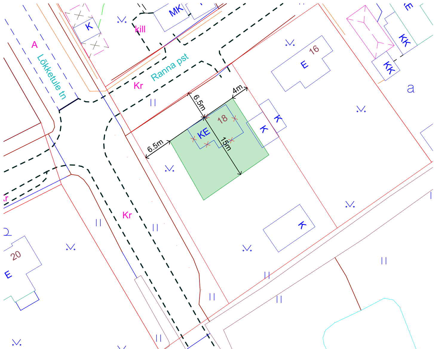
Lisa. Ehitusala skeem. Ranna pst 18 PTH-24-034
