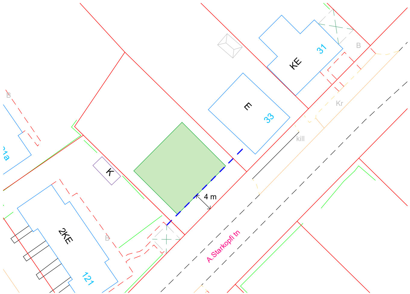
Lisa. A. Starkopfi tn 35 ehitusala skeem PTH-22-078
