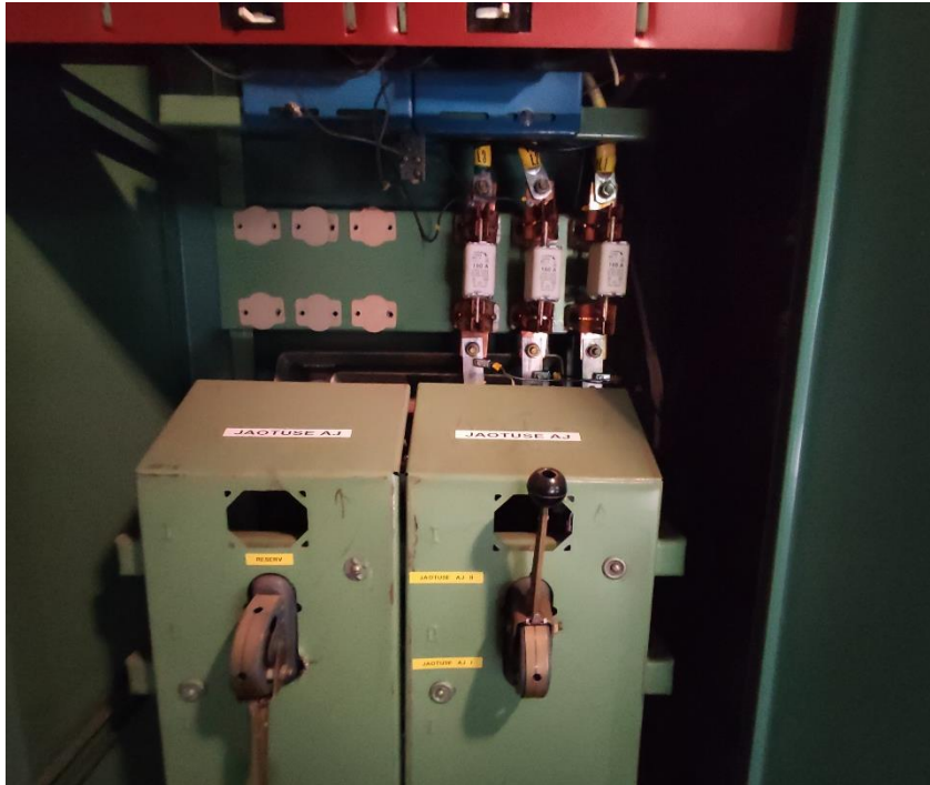
Joonis 2.11 Kilbiruumi olukord. Foto: Martin Kikas / TREA 20.07.2022 a.
