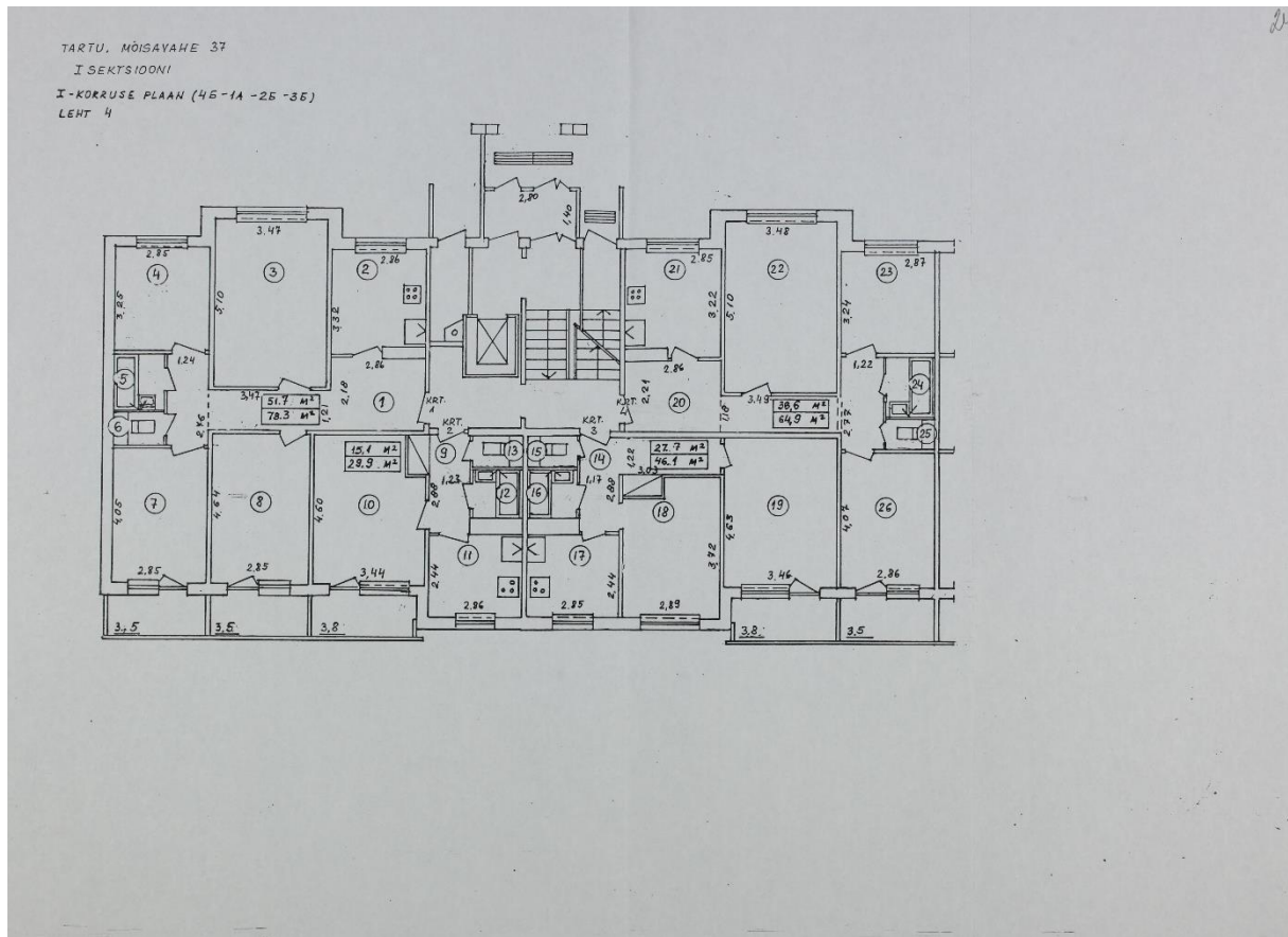
Joonis LISA1.0.3 I sektiooni I korruse plaan [3]
