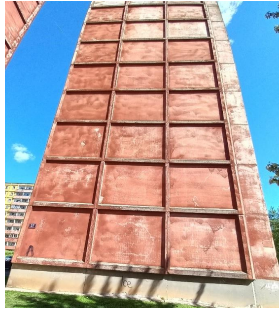
Joonis 2.4 Otsaseina- ja välisseina- ja akna detailid punasest hoonest. Foto: Martin Kikas / TREA 20.07.2022.a.
