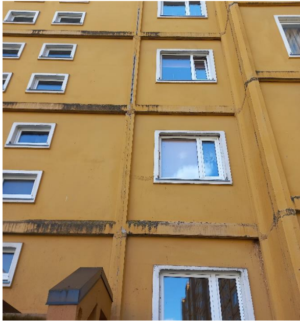
Joonis 2.3 Väli- ja välisseina- ja akna detailid kollasest hoonest. Foto: Tamur Tensing / TREA 20.07.2022 a.
