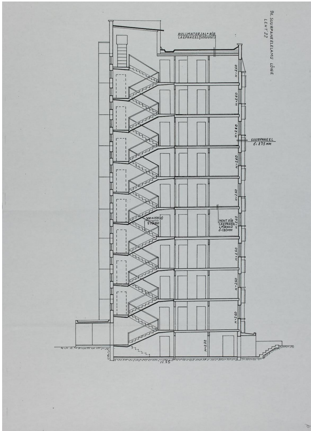
Joonis LISA1.0.1 Hoone lõige [3]
