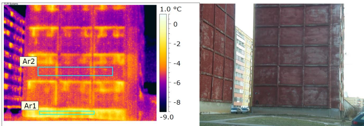
Joonis 1.3 Termokaamera ülesvõte otsaseinast [7]
