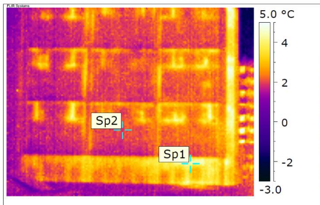
Joonis 1.4 Termokaamera ülesvõte otsaseinast [7]
