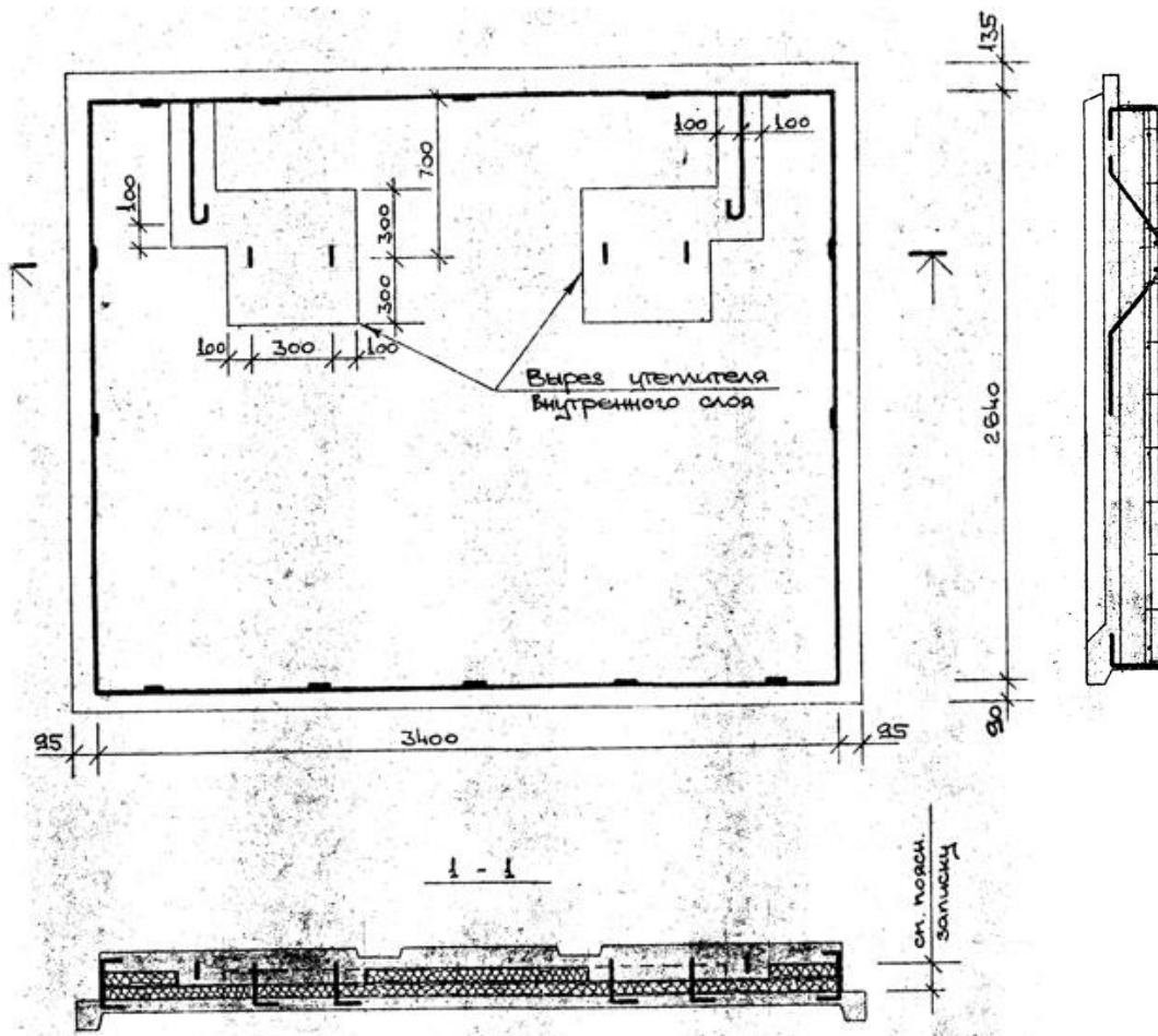
Joonis 1.5 Tüüpiline otsaseina raudbetoonpaneel [6]
