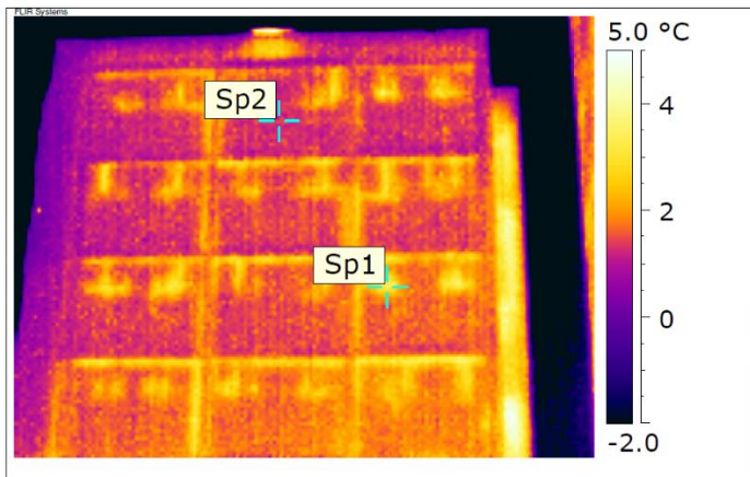
Joonis 1.3 Termokaamera ülesvõte otsaseinast [7]
