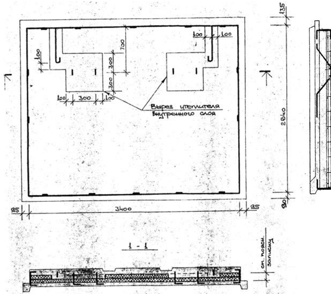
Joonis 1.4 Tüüpiline otsaseina raudbetoonpaneel [4]
