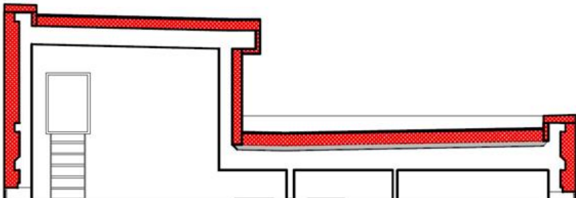
Joonis 3.1 Katuse tehniline lahendus, variant 1 [10]
