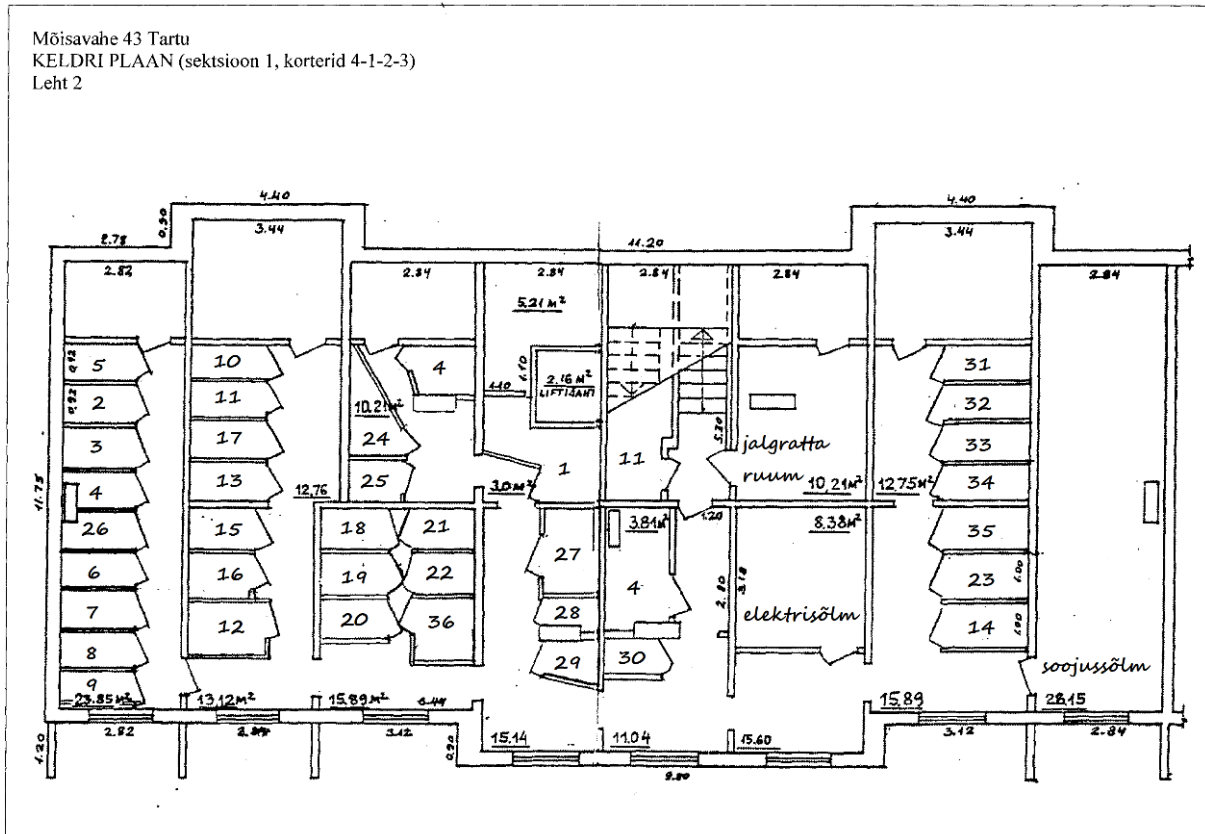
Joonis LISA1.0.1 | seksiooni keldrikorruse plaan [7]
