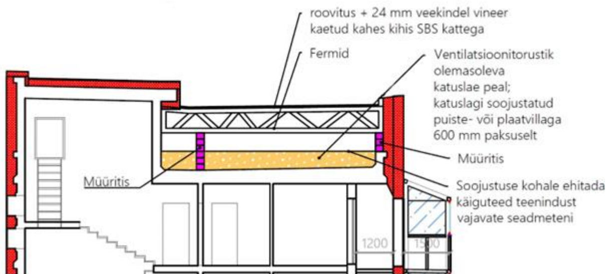
Joonis 3.3 Katuse tehniline lahendus, variant 3 [10]
