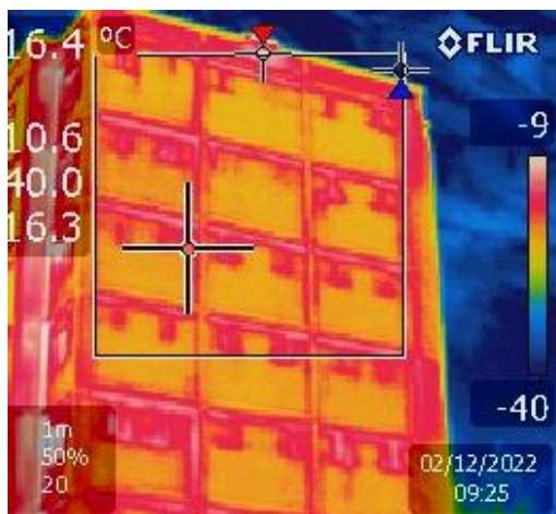
Joonis 1.3 Termokaamera ülesvõtte otsaseinast. Foto: Ain Konsap / TREA 02.12.2022
