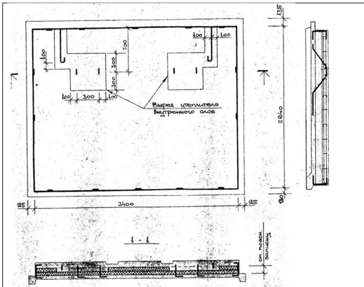
Joonis 1.4 Tüüpiline otsaseina raudbetoonpaneel [5] [5]
