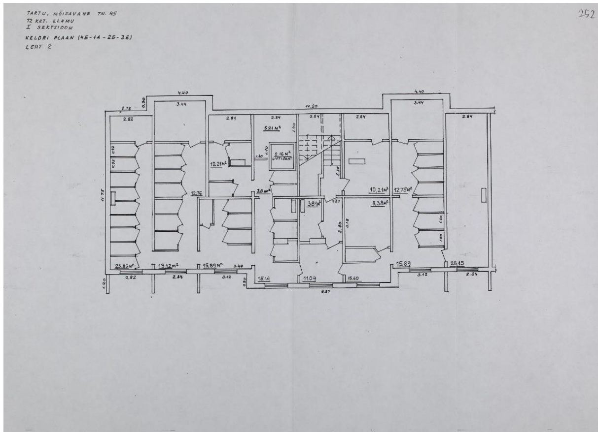
Joonis LISA1.0.2 I sektsiooni keldrikorruse plaan [3]
