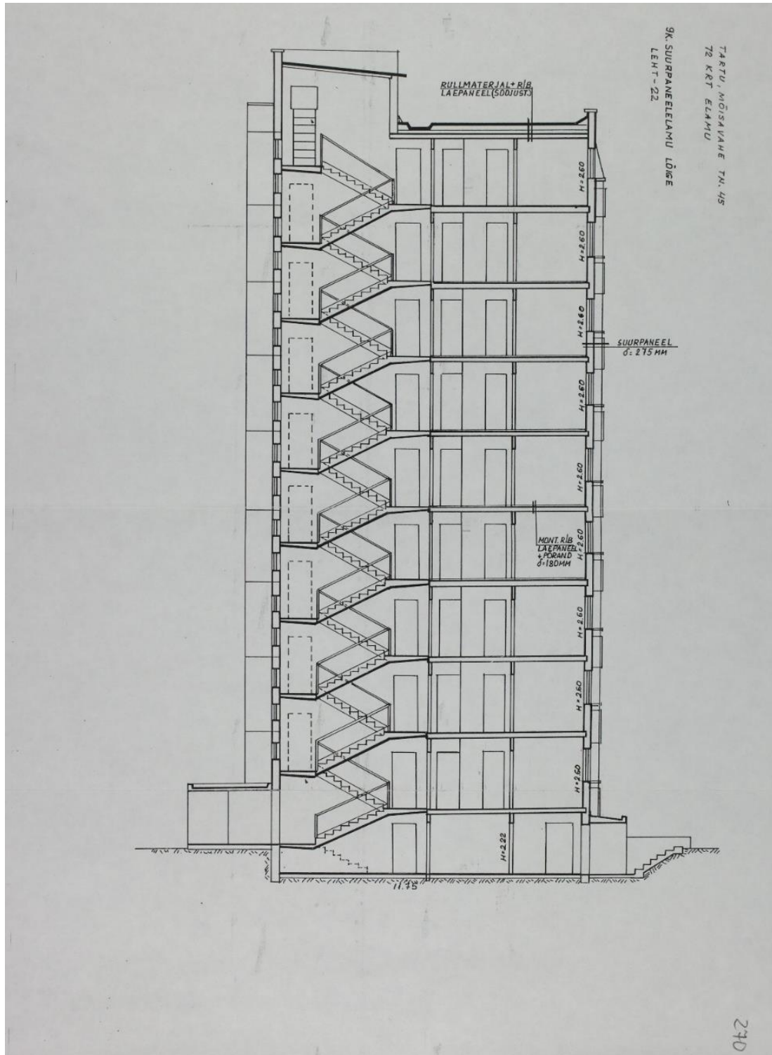
Joonis LISA1.0.1 Hoone lõige [4]
