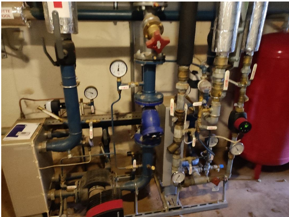
Joonis 2.7 Soojussõlme olukord. Foto: Martin Kikas / TREA 19.07.2022 a
