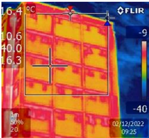
Joonis 1.3 Termokaamera ülesvõte Mõisavahe 43, Tartu otsaseinast. Foto: Ain Konsap / TREA 02.12.2022
