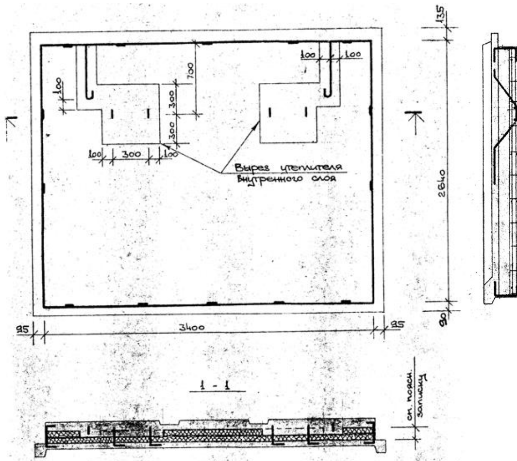
Joonis 1.4 Tüüpiline otsaseina raudbetoonpaneel [5]
