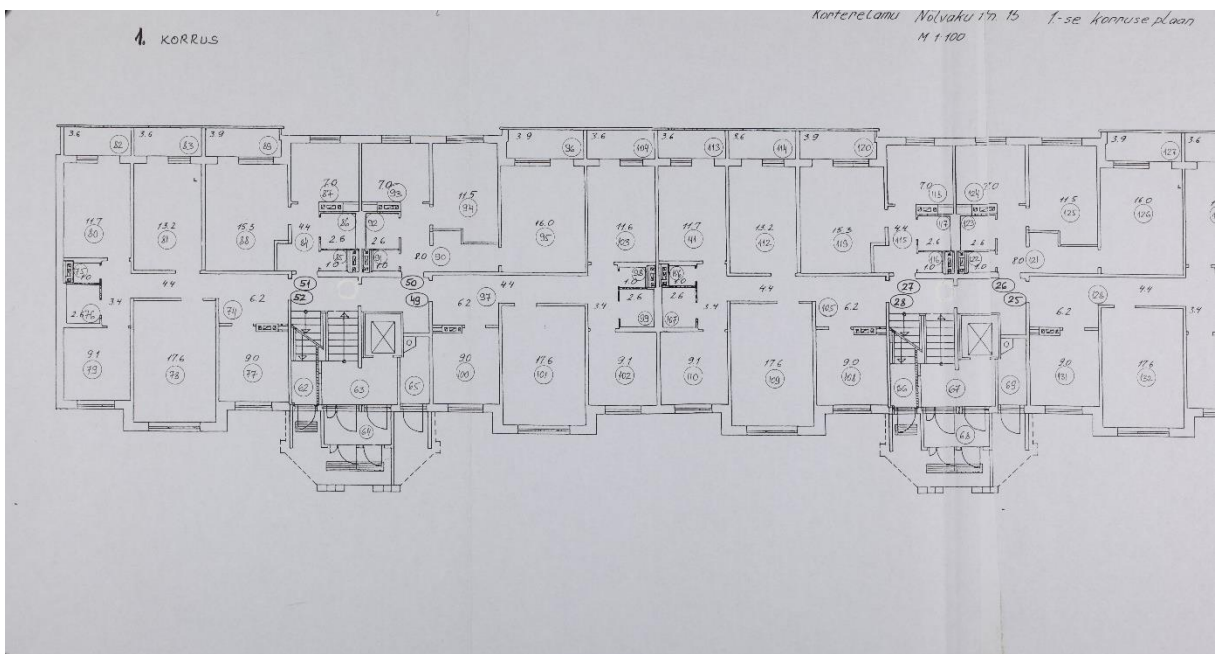
Joonis LISA1.0.2 I sektsiooni I korruse plaan [3]
